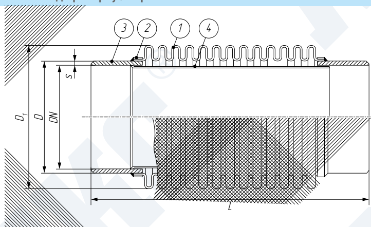
КСО ARM под приварку / чертёж
